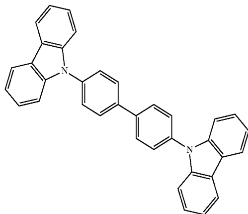
CBP
